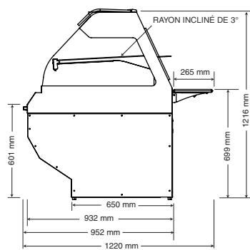
ED2SYS-96/2S Vue de côté
