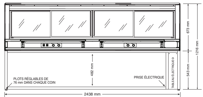
ED2SYS-96/2S Vue arrière
